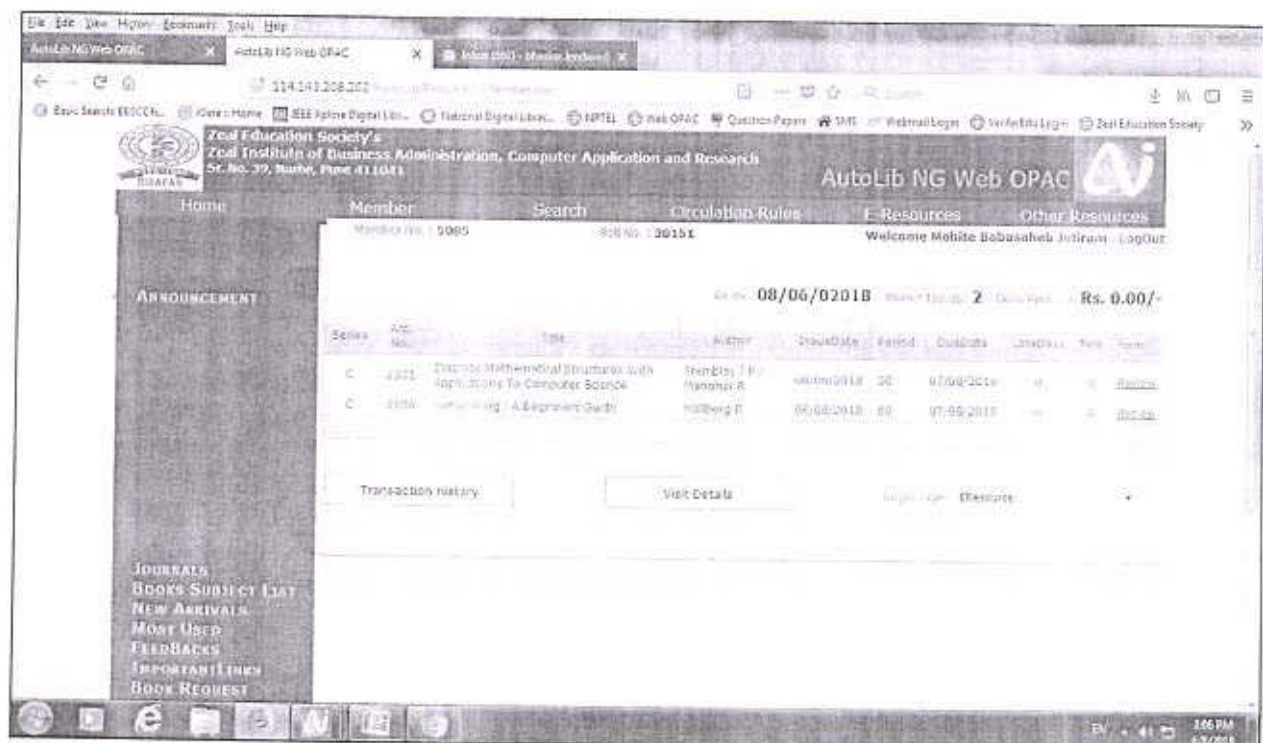
Photo 4. Web OPAC
